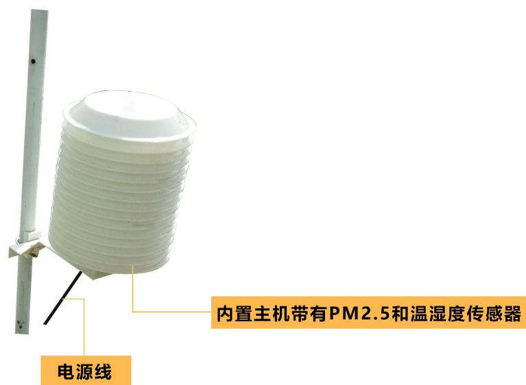
图三 RA0716Y 屏蔽罩内接内接 PM2.5 和温湿度 Sensor (以实物为准)
